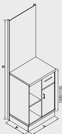
SCAFFALE MACCHINA CAFFE' CON STRUTTURA IN TUBOLARE DI ALLUMI- NIO-
