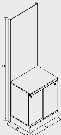
SCAFFALE CON BASE H770 SHELF WITH BASE H770 - MEUBLE AVEC BASE H770 REGAL MIT BASELEMENT H770
