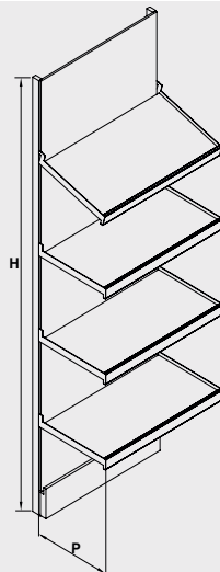
SCAFFALE CON RIPIANO BASE E MENSOLE SHELVES RACK - MEUBLE AVEC ETAGERE - REGAL MIT ABLAGE
